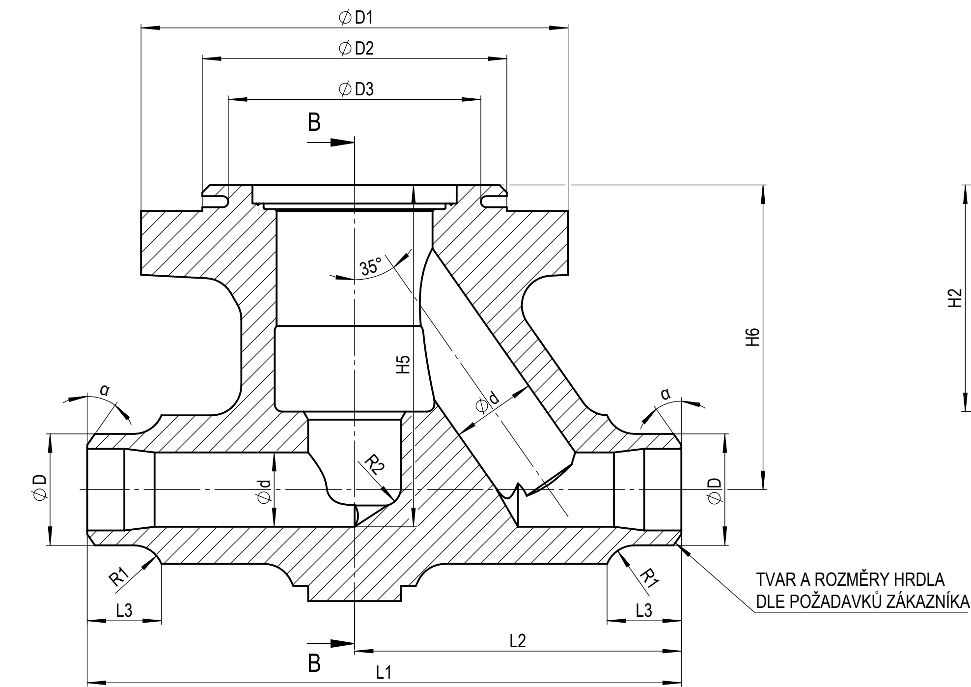
ŘEZ A-A
