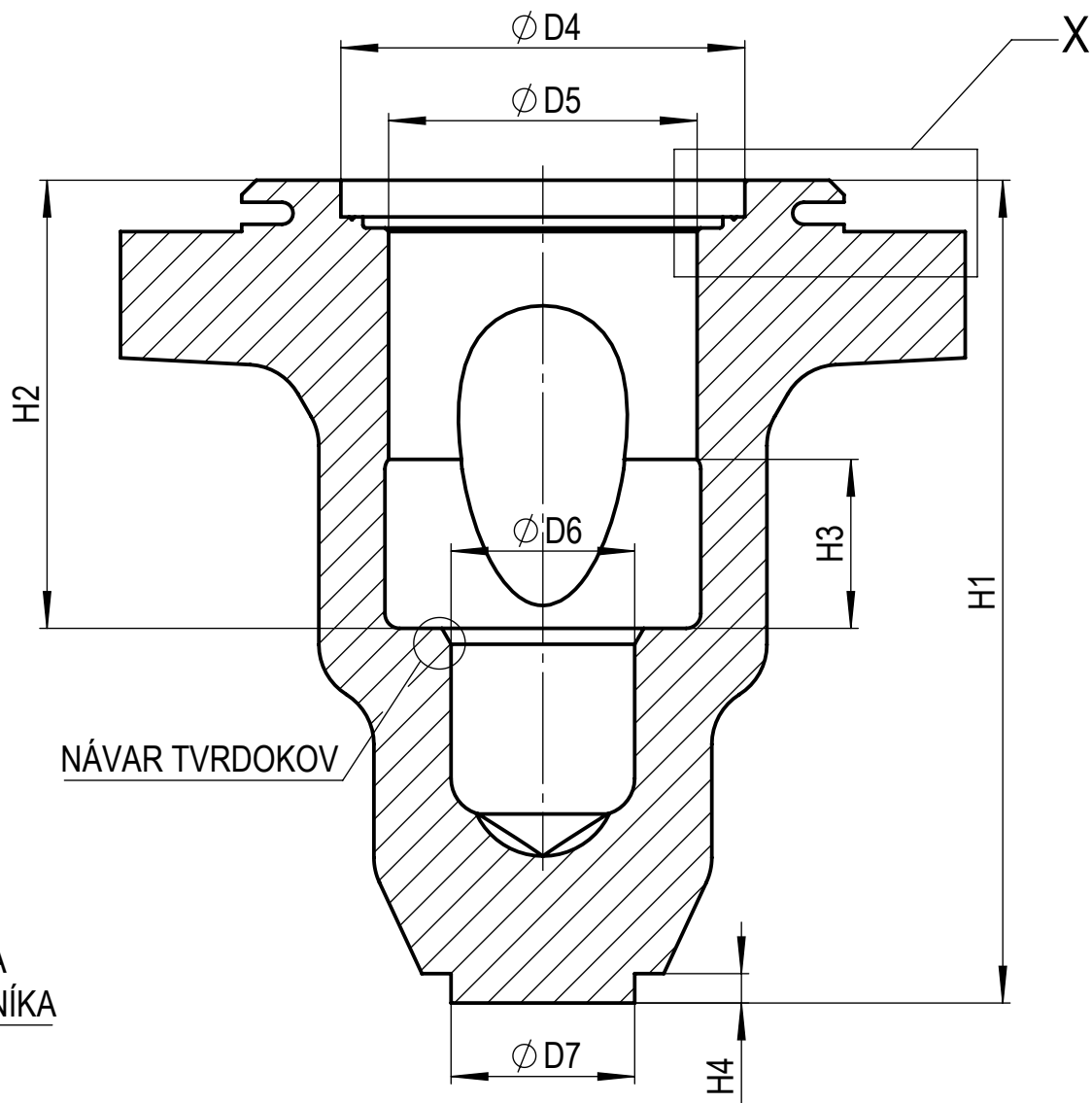
ŘEZ B-B
