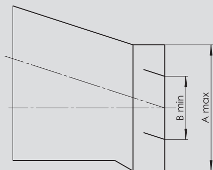
Neobrobené přivařovací konce
