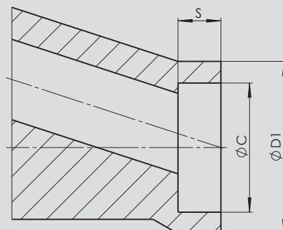
Socket weld konce
